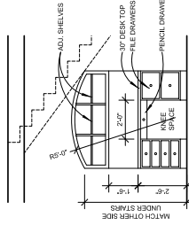
INTERIOR ELEVATION SCALE: 3/8" = 1'-0"
